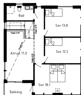
ÖVERPLAN
