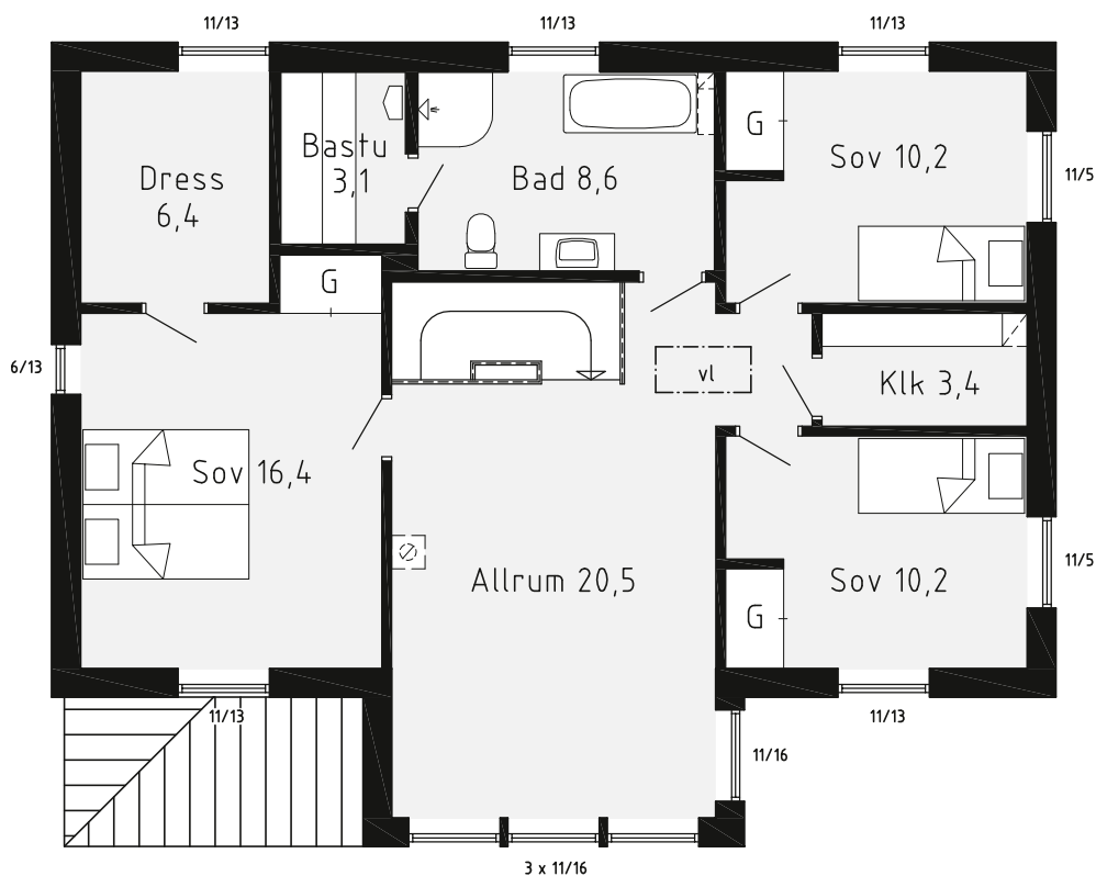
ÖVERPLAN
