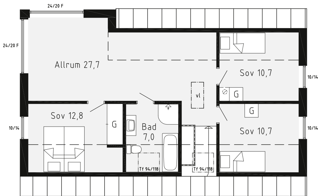
ÖVERPLAN
