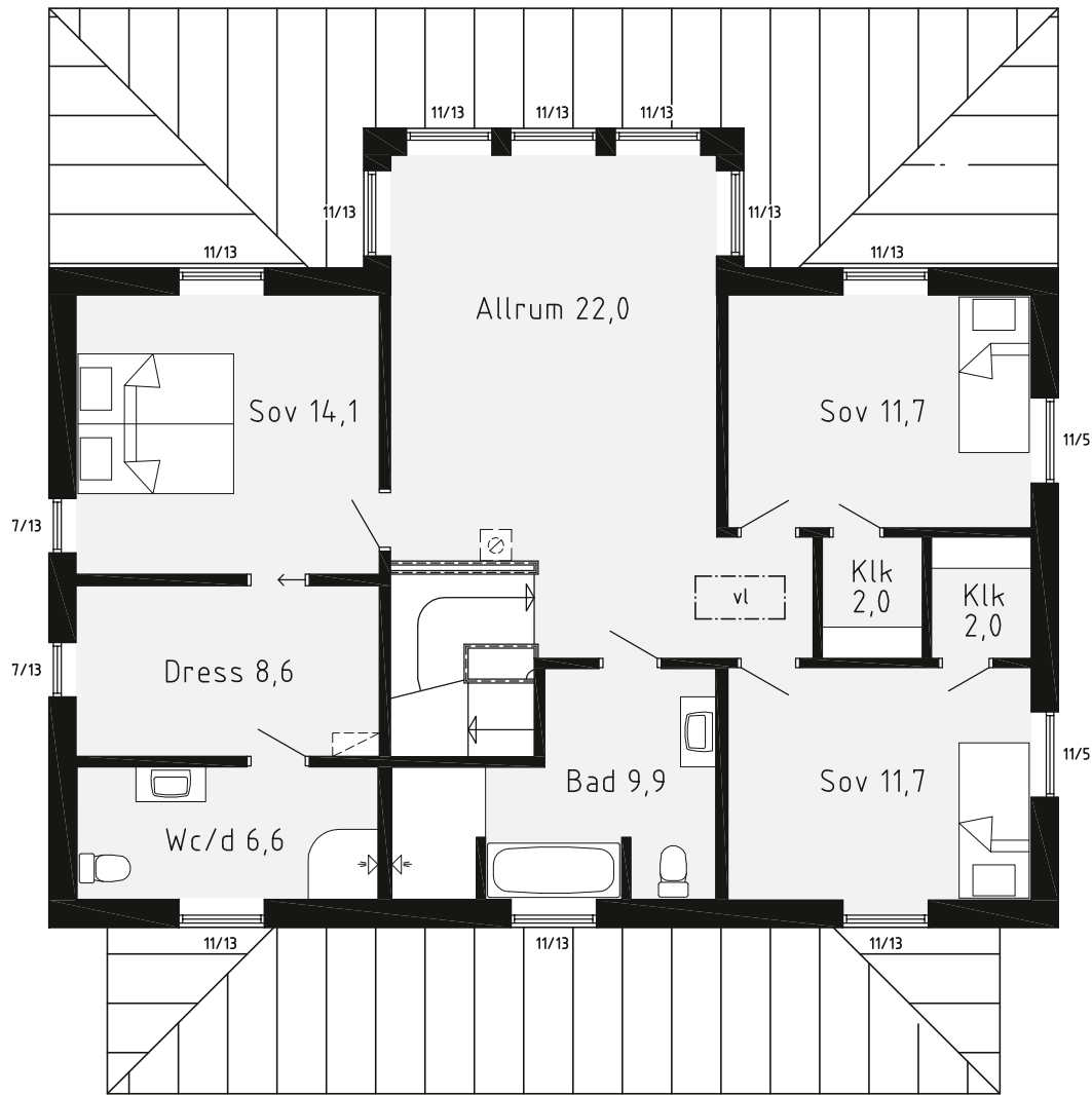
ÖVERPLAN
