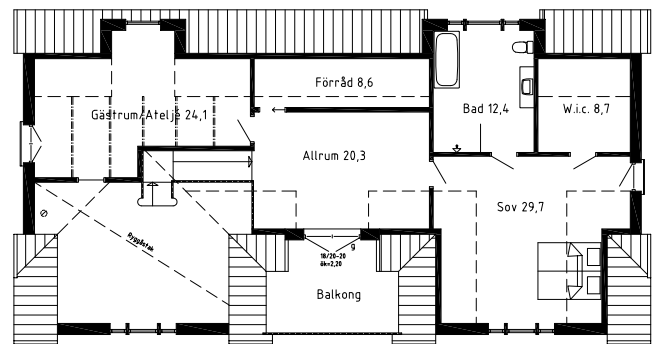
ÖVERPLAN
