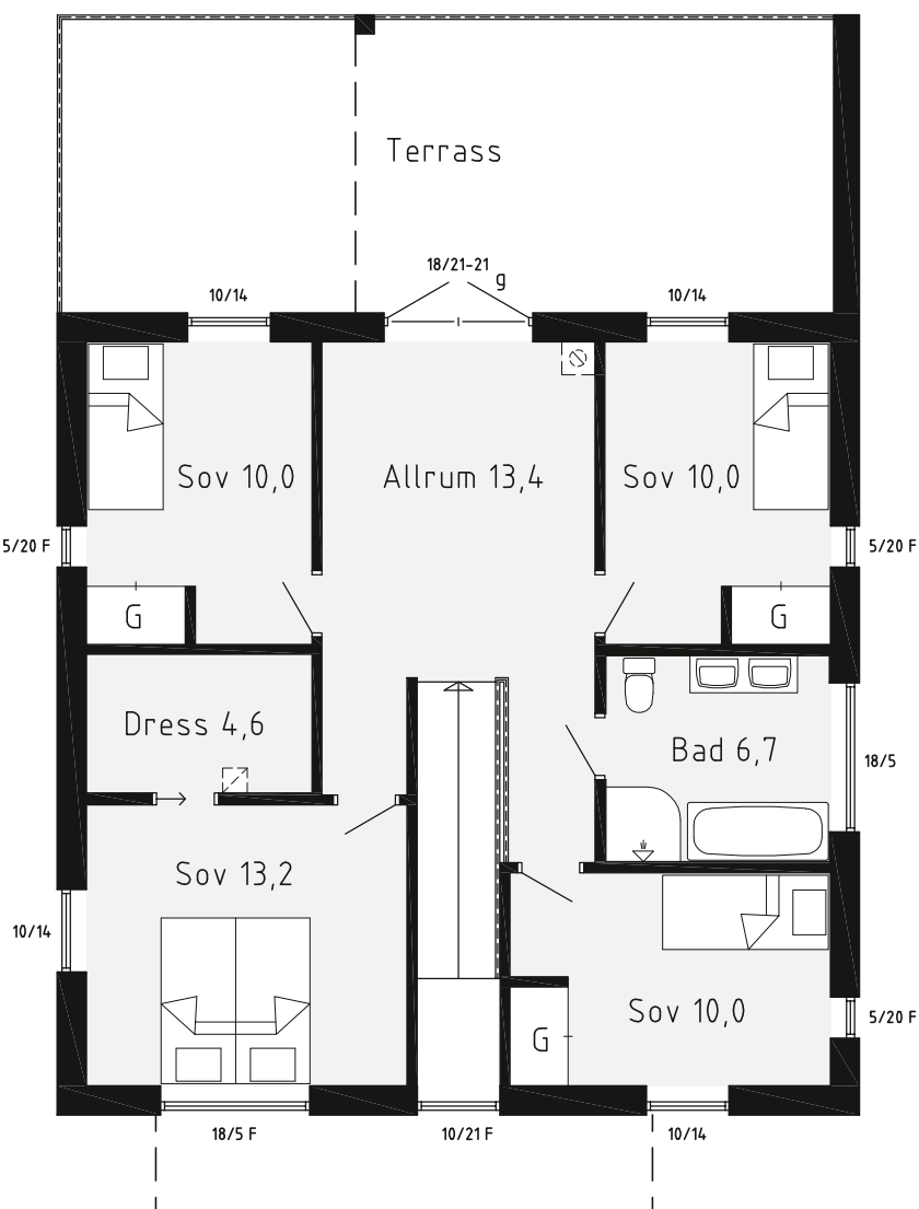
ÖVERPLAN
