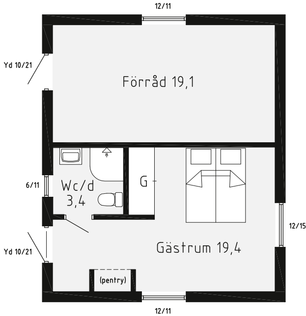
SIDOBYGGNADER
