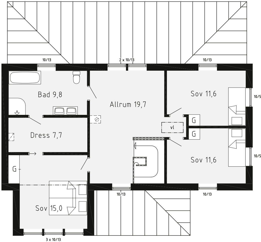
ÖVERPLAN
